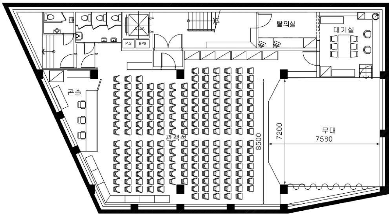
지하 1층 평면도
