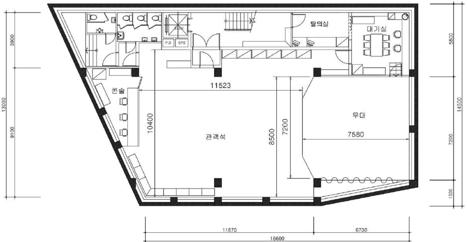
지하 1층 평면도
